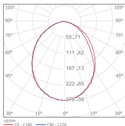
MDL-DL35R08W-03
