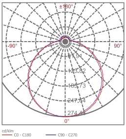
MDL-CL36W
