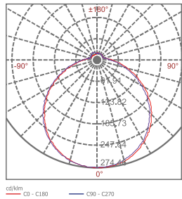
MDL-CLR24W-03
