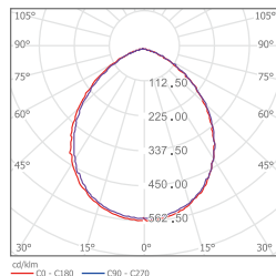
MDL-DL06R20W-04
