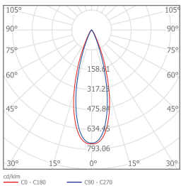
MDL-TL3L09W
