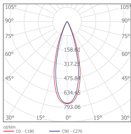
MDL-TL242TW09W
