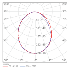
MDL-DL04S08W
