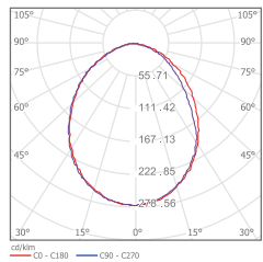
MDL-DLM04S08W
