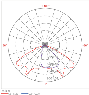
MDL-SLW150W
